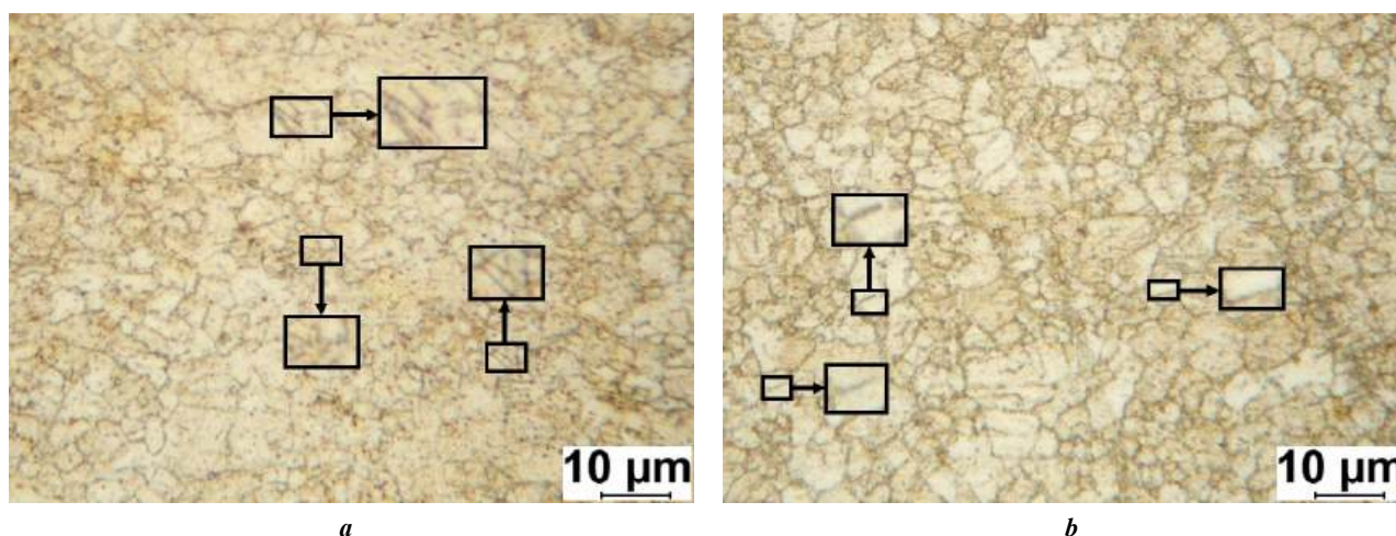
Рис. 6. Микроструктура латуни Л68 после ротационной ковки при комнатной температуре и последующего отжига в течение 30 мин (а) и 2 ч (б). Стрелки указывают на двойники Fig. 6. Microstructure of L68 brass after rotary swaging at room temperature and subsequent annealing for 30 min (a) and 2 h (b). Arrows indicate twins
