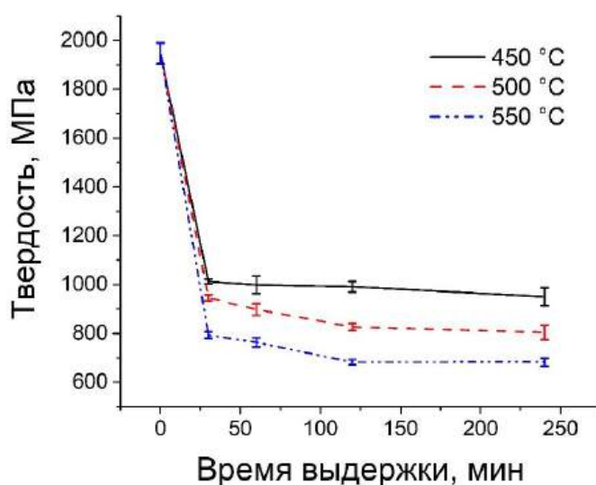
Рис. 4. Зависимость твердости латуни Л68 после ротационной ковки от температуры и времени нагрева Fig. 4. Dependence of the hardness of L68 brass after rotary swaging on the temperature and heating time
