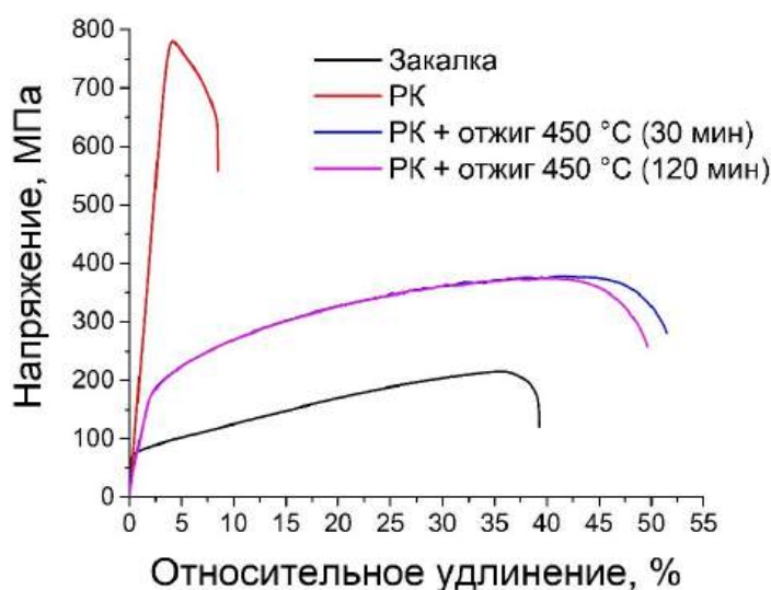
Рис. 5. Кривые растяжения латуни Л68 в различных состояниях Fig. 5. Stress-strain curves of L68 brass in different states
