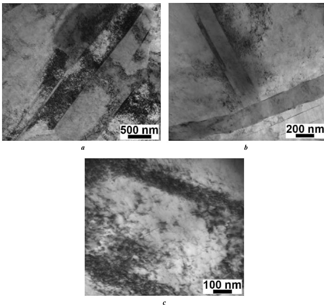
Рис. 2. ПЭМ-изображения латуни Л68 после ротационной ковки: структура сплава при увеличениях \times 25\,000 (a), \times 50\,000 (b) и \times 100\,000 (c) Fig. 2. TEM images of L68 brass after rotary swaging: alloy structure at magnifications of \times 25,000 (a), \times 50,000 (b) and \times 100,000 (c)
