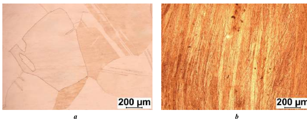
Рис. 1. Микроструктура латуни Л68 в закаленном состоянии (а) и после ротационнойковки при комнатной температуре (б)
