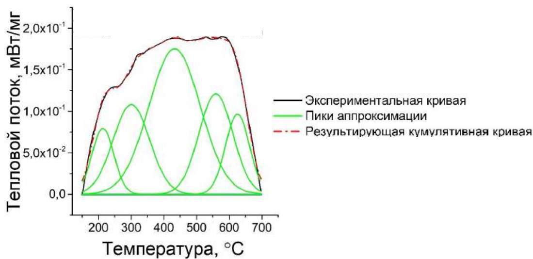
Рис. 3. Зависимость теплового потока от температуры нагрева для латуни Л68 после ротационной ковки Fig. 3. Dependence of heat flow on heating temperature for L68 brass after rotary swaging
