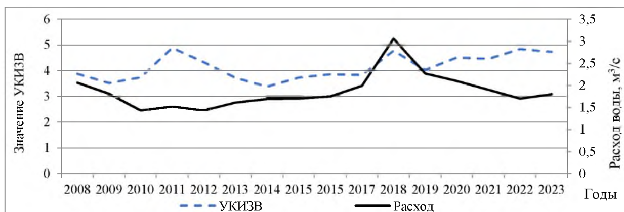
Рис. 4. Динамика удельного комплексного индекса загрязненности воды в створе Белгородского водохранилища
