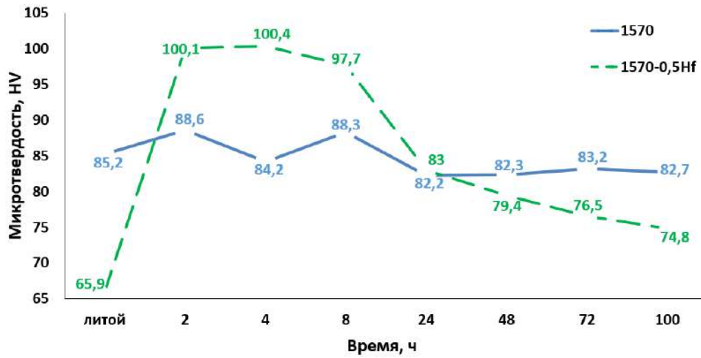
Рис. 1. Изменение микротвердости при отжиге 440 °С Fig. 1. Change in microhardness during 440 °C annealing
