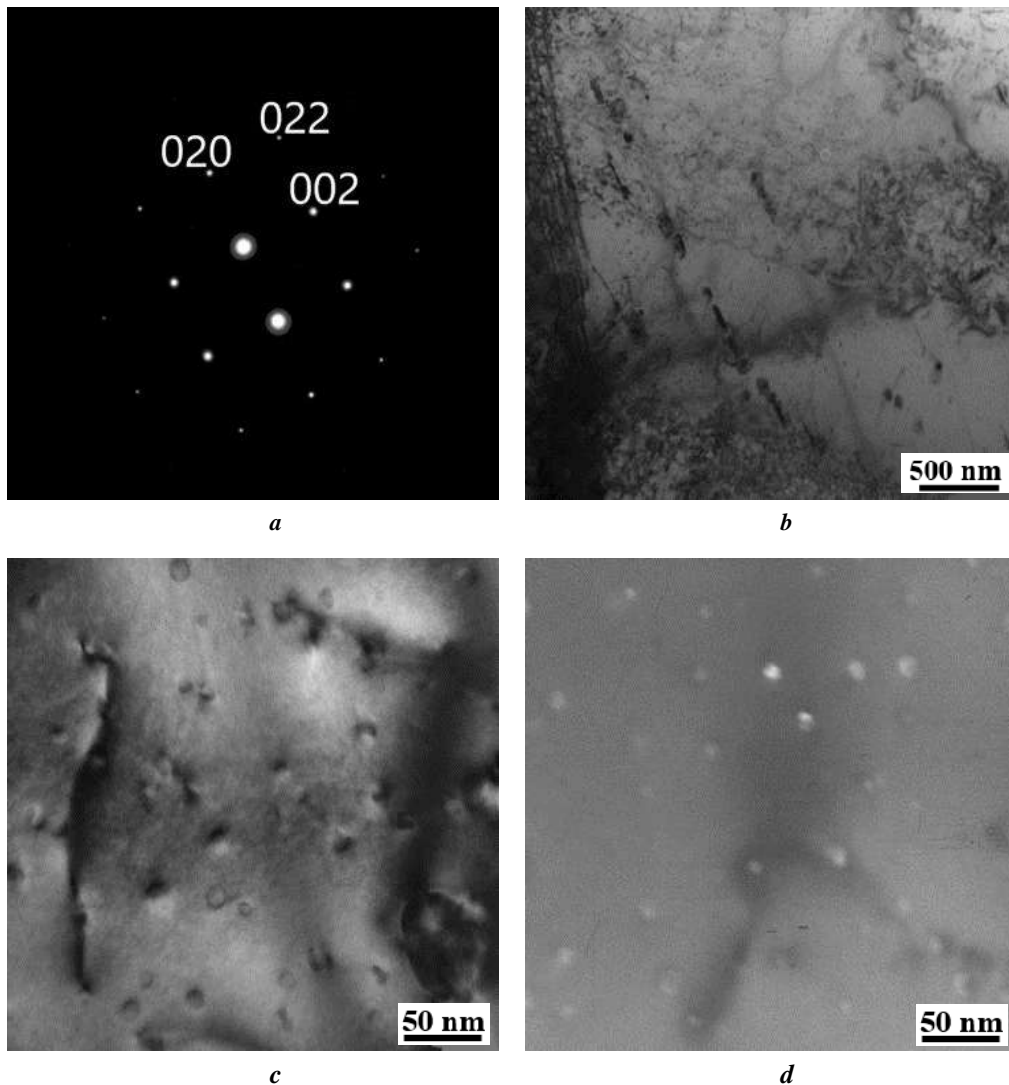
Рис. 4. Тонкая структура сплава 1570–0,5Hf при отжиге при 440 °С длительностью 4 ч: a – микродифракция в оси зоны [001]; b – светлое поле, ×20 000; c, d – темное поле, ×200 000 Fig. 4. Fine structure of 1570–0.5Hf alloy during 440 °C annealing with a duration of 4 h: a – microdiffraction in the zone axis [001]; b – bright field, ×20,000; c, d – dark field, ×200,000
