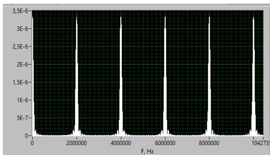
Рис. 5. Идеальная передискретизация Fig. 5. Idealized subsampling
