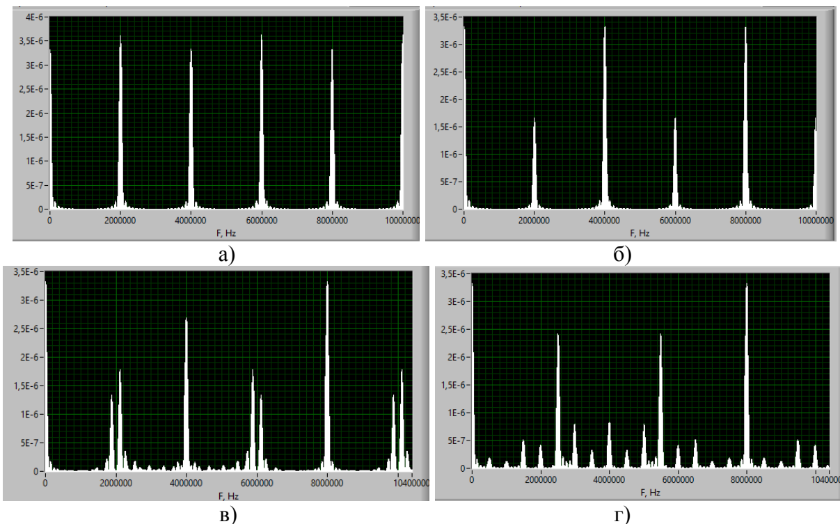
Рис. 6. Воздействие детерминированного джиттера: а) 100 Гц; б) 1кГц; в) 100 кГц; г) 500 кГц Fig. 6. The impact of deterministic jitter: a) 100 Hz; б) 1kHz; в) 100 kHz; г) 500 kHz
