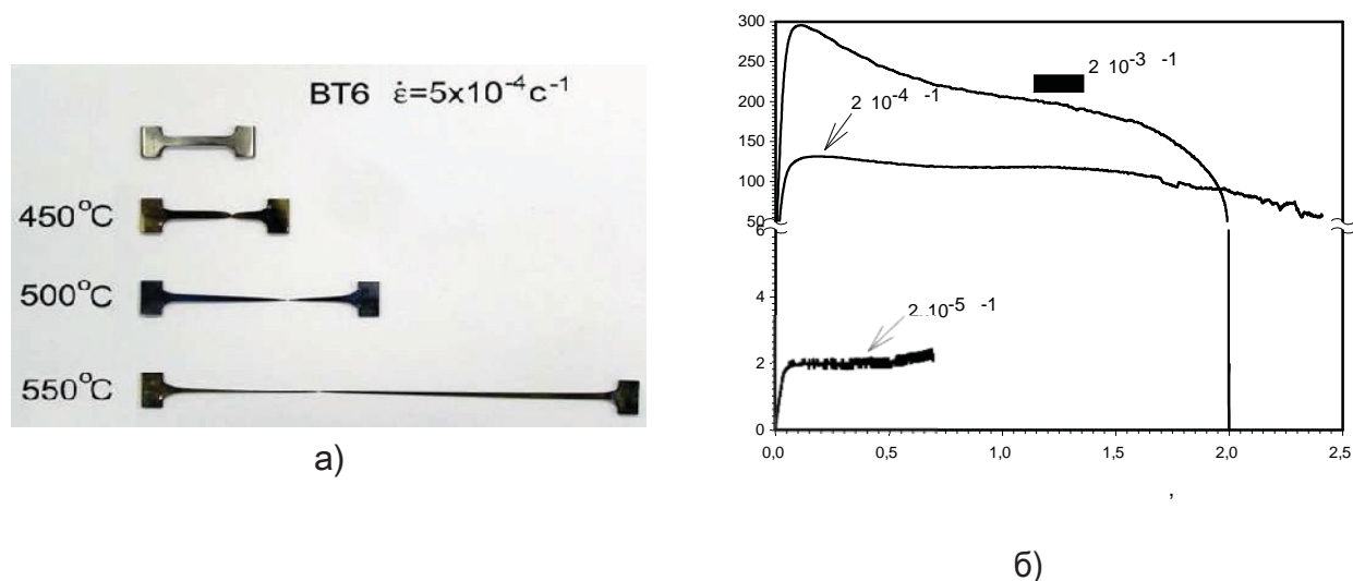
Рис. 3. Вид образцов сплава ВТ6 с УМЗ структурой после деформации при разных температурах испытания и скорости 5 \times 10^{-4} \text{с}^{-1} (а); кривые истинные напряжения течения – истинная деформация для сплава ВТ6 полученные при T=550^\circ\text{C} и разных скоростях деформации (б).
