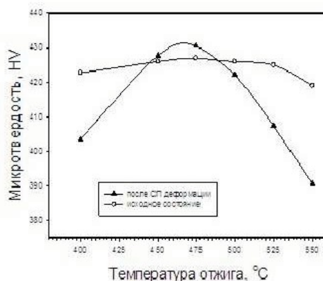
Рис. 7. Изменение микротвердости УМЗ титанового сплава ВТ6 в зависимости от температуры отжига, t=2 ч, после сверхпластической деформации при скорости 2 \times 10^{-4} \text{ с}^{-1} и в исходном состоянии.
