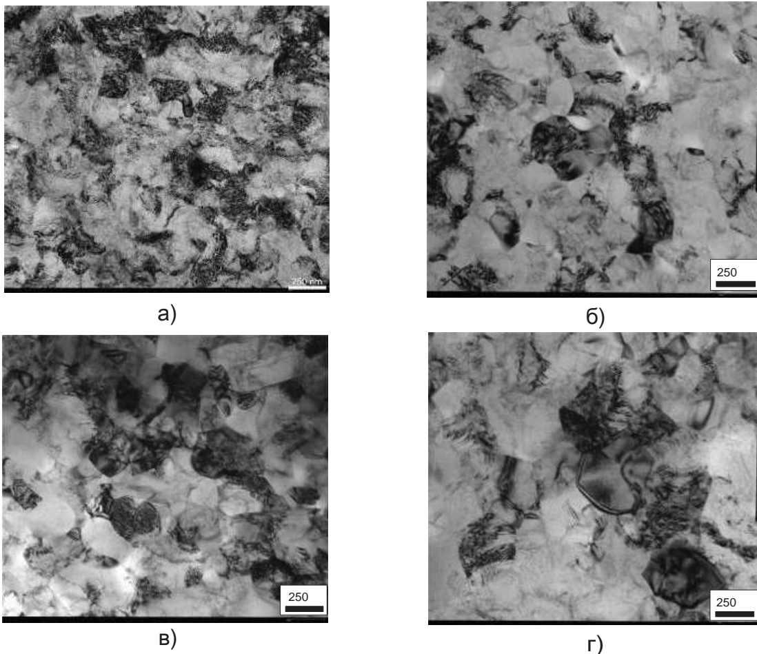
Рис. 6. Микроструктура сплава ВТ6 в исходном состоянии (а) и подвергнутого сверхпластической деформации при температуре T=550^{\circ}\text{C} и скоростях деформации \dot{\epsilon}=5 \times 10^{-3} \text{c}^{-1} (б); \dot{\epsilon}=2 \times 10^{-4} \text{c}^{-1} (в); \dot{\epsilon}=5 \times 10^{-5} \text{c}^{-1} (г).
