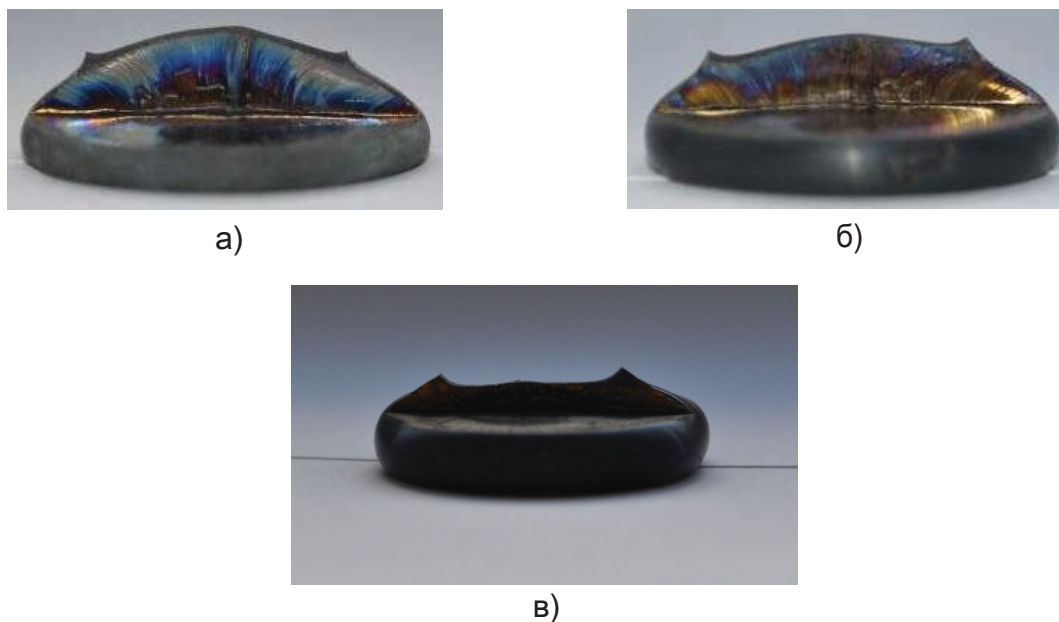
Рис. 5. Заполняемость формы, определенная в ходе осадки на щелевом штампе УМЗ сплава ВТ6 со степенью деформации \epsilon=90\% , \dot{\epsilon}=2 \times 10^{-5} \text{с}^{-1} (а); \dot{\epsilon}=2 \times 10^{-4} \text{с}^{-1} (б); \dot{\epsilon}=5 \times 10^{-3} \text{с}^{-1} (в).
