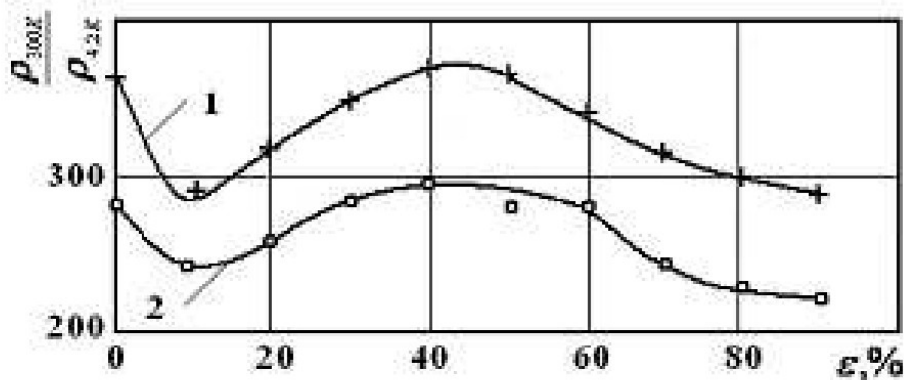
Рис. 2. Зависимость относительного остаточного электросопротивления для меди MB (1) и MMB (2) от величины предварительной деформации после отжига образцов при 550°С, 1 час.
