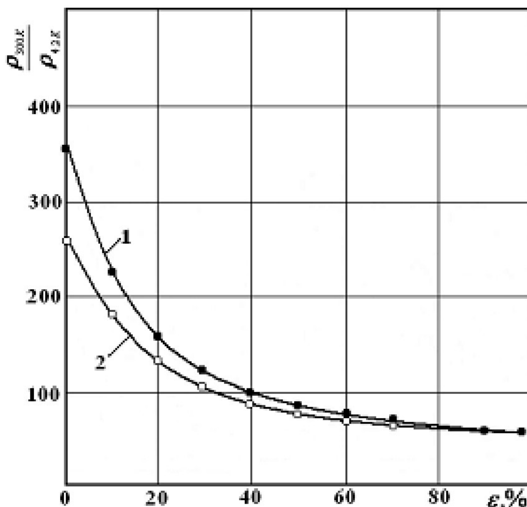
Рис.1. Зависимость относительного остаточного электросопротивления от величины предварительной деформации для меди MB (1), MMB (2).
