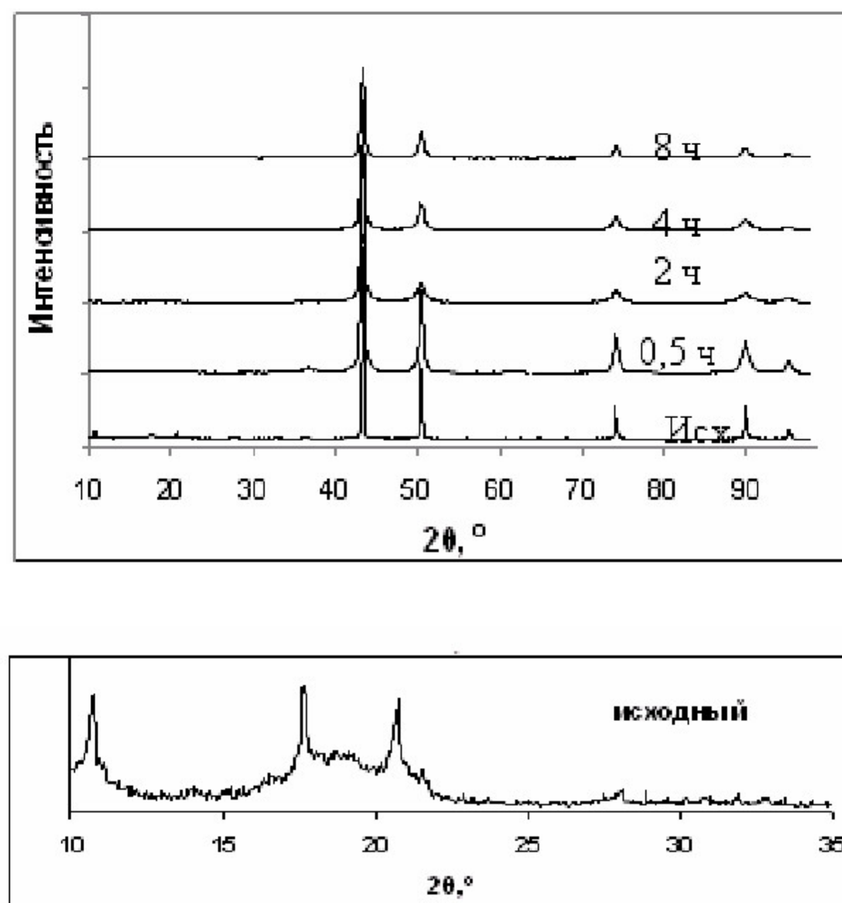
Рис. 1. Дифрактограммы смеси Cu-25%С60/70 после различных времен МА.
