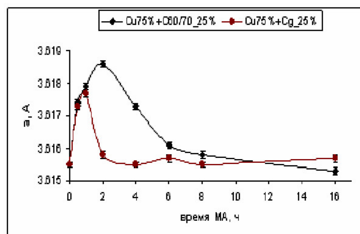
Рис. 2. Изменение параметра решетки меди в зависимости от времени МА.
