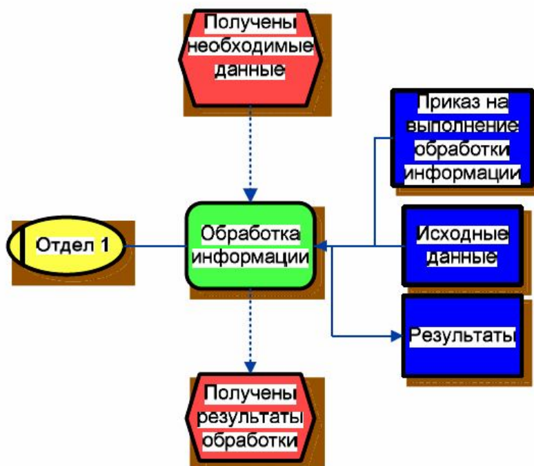
Рис. 2. Пример eEPC-диаграммы
