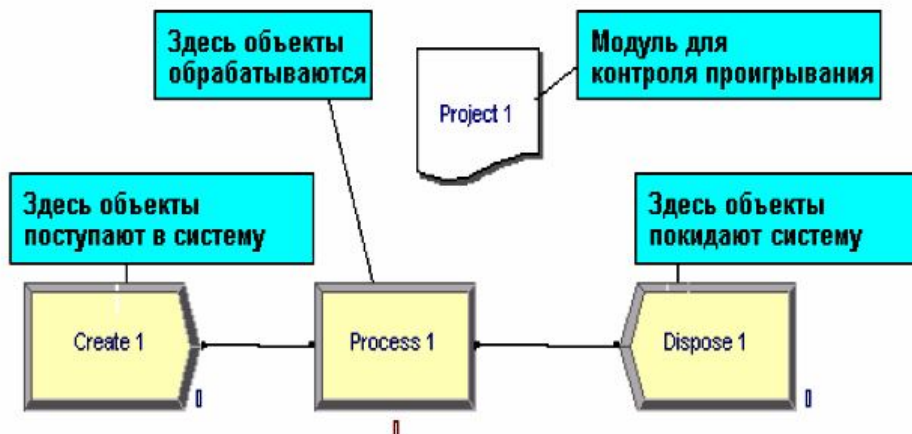
Рис. 3. Простейшая имитационная модель в Arena
