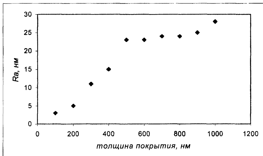
Рис. 4. Зависимость степени шероховатости углеродного конденсата от его толщины.
