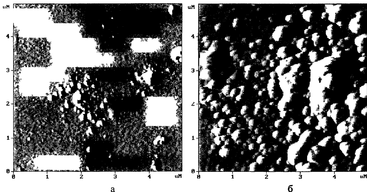
Рис. 1. Топография углеродного конденсата толщиной 100 нм (а) и 1000 нм (б), размер поверхности сканирования 5 мкм × 5 мкм
