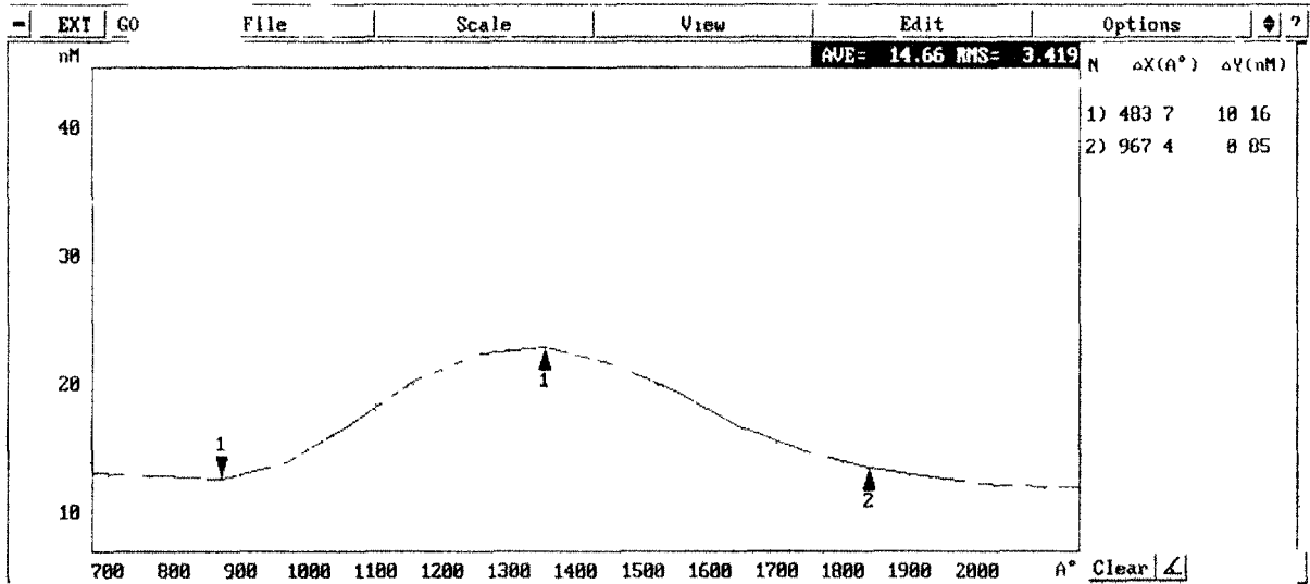
Рис. 5. Профилограмма отдельного микровыступа на поверхности углеродного конденсата толщиной 100 нм
