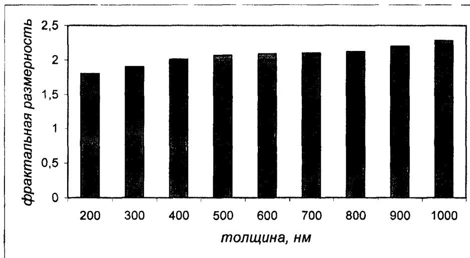
Рис. 6. Диаграмма зависимости фрактальной размерности поверхности углеродного покрытия от его толщины.
