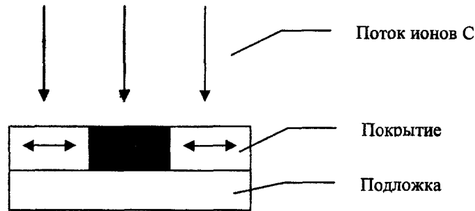
Рис. 7. Схема, поясняющая процесс формирования углеродного покрытия на подложке.
