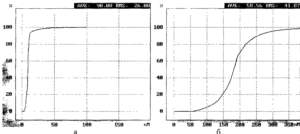
Рис. 3 а, б. Зависимости распределения плотности объектов в процентном соотношении от их высоты для углеродных конденсатов толщиной 100 и 1000 нм соответственно.
