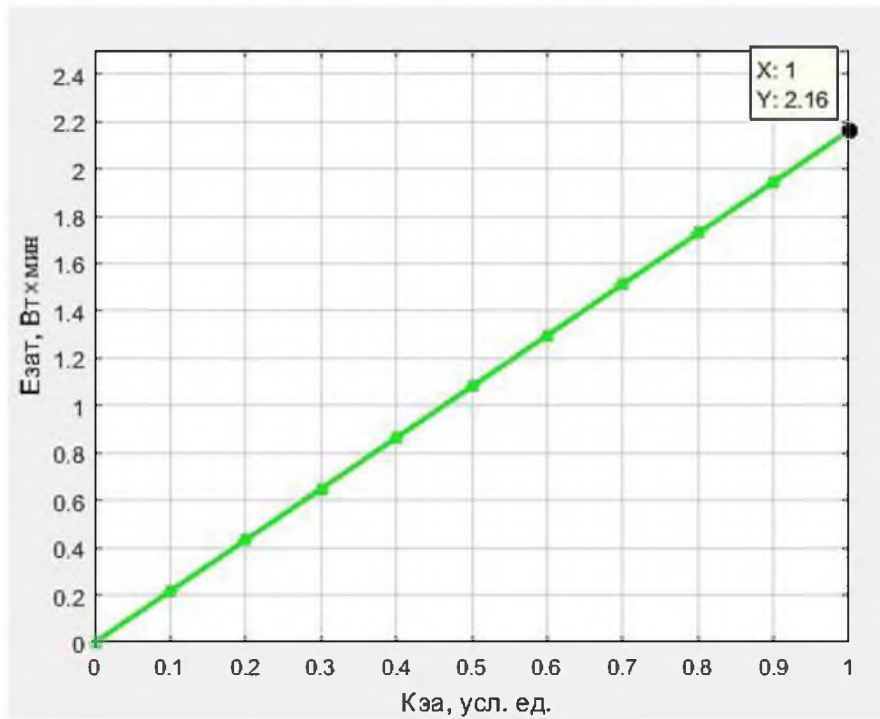
Рис. 5. График зависимости расходуемой энергии БСС ( E_{зат} ) от величины K_{ЭА}
