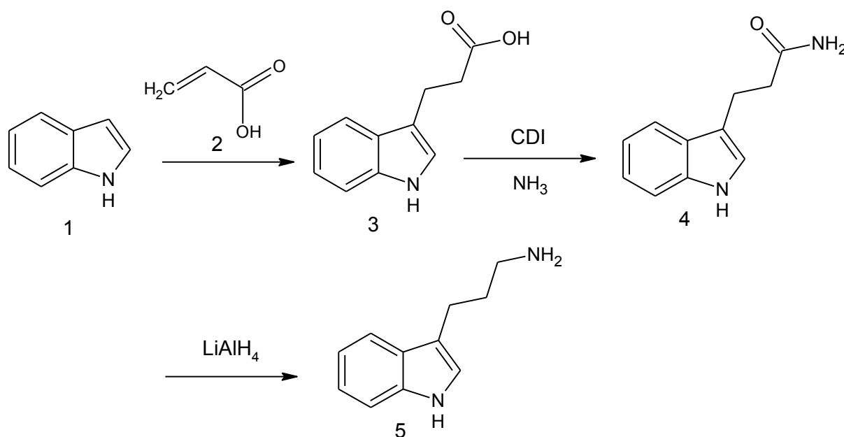
Рис. 1.1. Синтез гомотриптамина с использованием акриловой кислоты
