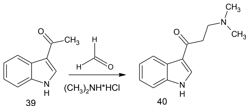
Рис. 1.20. Синтез 3-кето-3-индолил-N,N-диметилпропанамина
