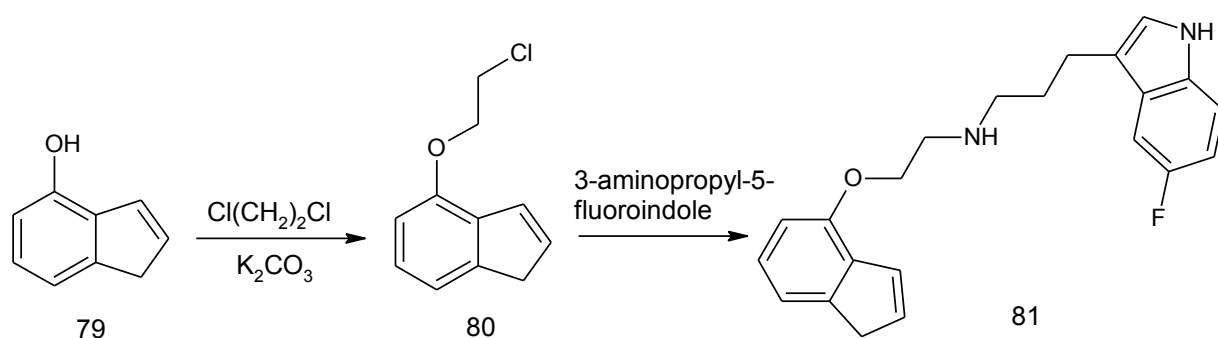
Рис. 1.33. Синтез N-производного 5-фторгомтриптамина
