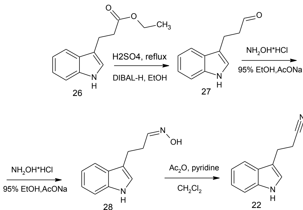
Рис. 1.12. Синтез индолилпропионатнитрила на основе сложного эфира
