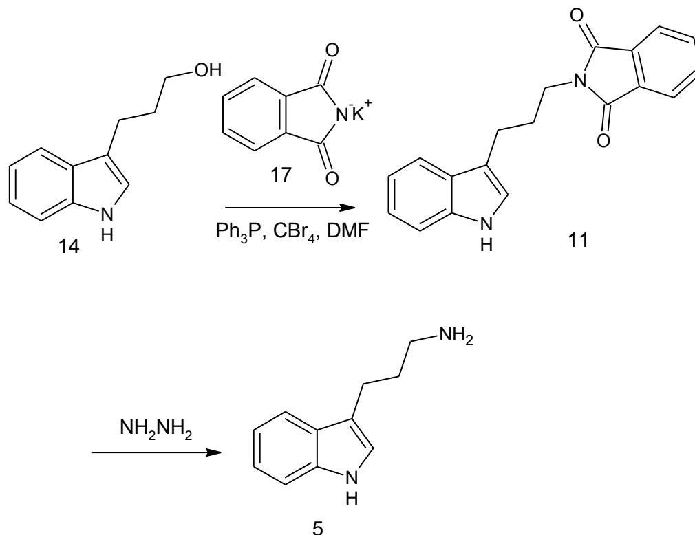
Рис. 1.7. Синтез гомотриптамина с использованием фталимида калия
