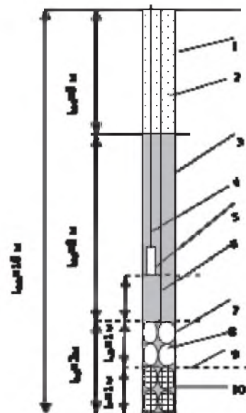
Рис. 5. Общий вид скважинного заряда ВВ: 1 – буровая скважина; 2 – песчаная забойка; 3 – основной заряд ВВ; 4 – детонирующий шнур; 5 – детонатор; 6 – шнур для крепления гирлянды; 7 – рукав из полиэтилена; 8 – воздушная емкость; 9 – уровень; 10 – кумулятивный отражатель
